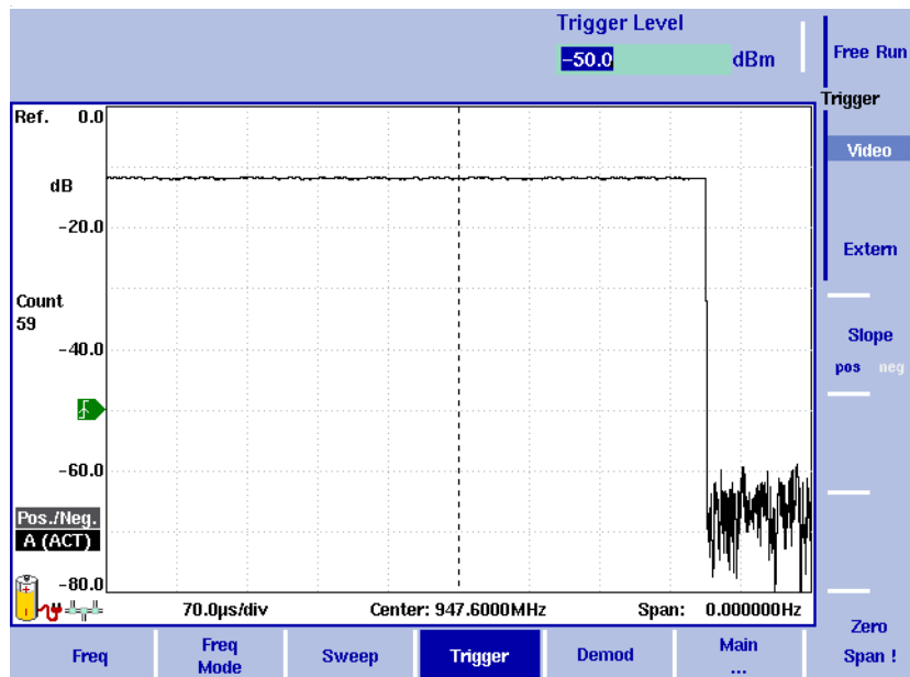
Abbildung 17 Ausgelöste Messung (im Zeitbereich)
