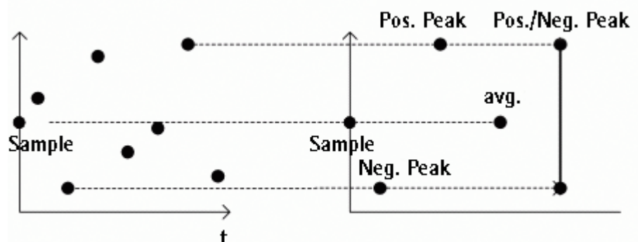
Abbildung 20 Trace-Detektoren
