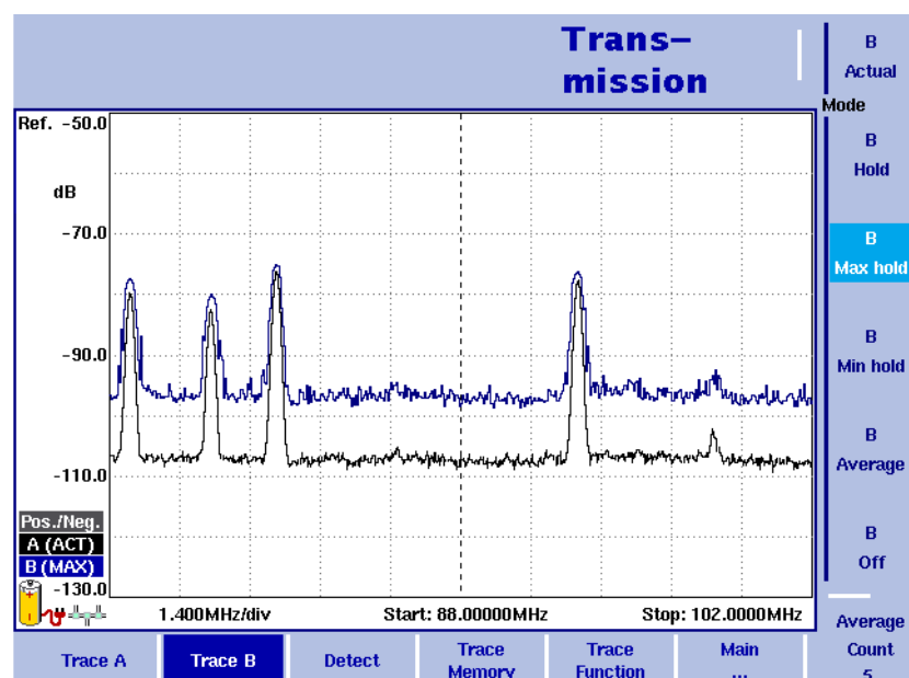
Abbildung 36 Beispiel für zwei Traces
