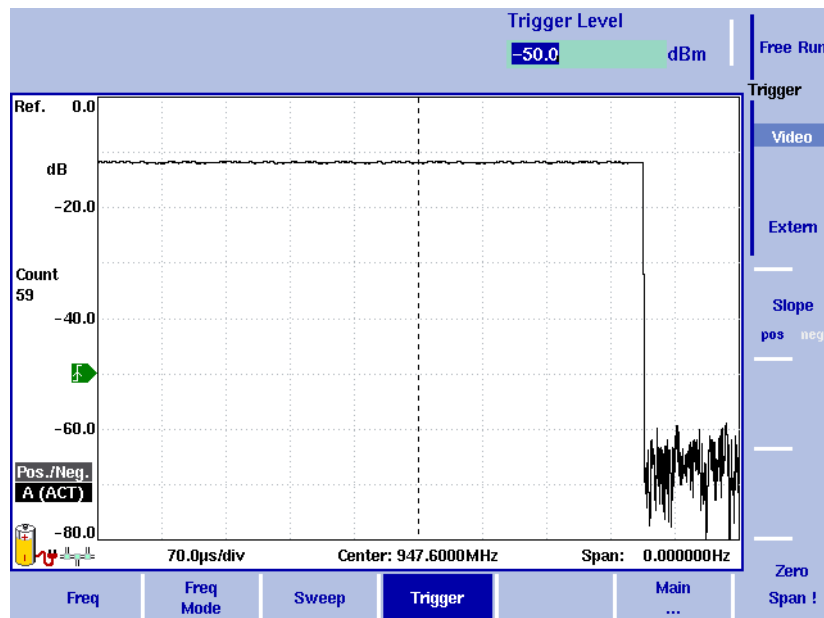
Abbildung 35 Ausgelöste Messung (im Zeitbereich)
