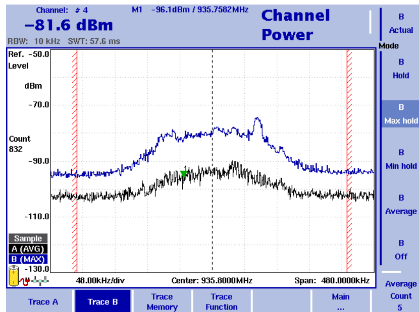
Abbildung 25 Beispiel für zwei Traces im Modus Channel Power
