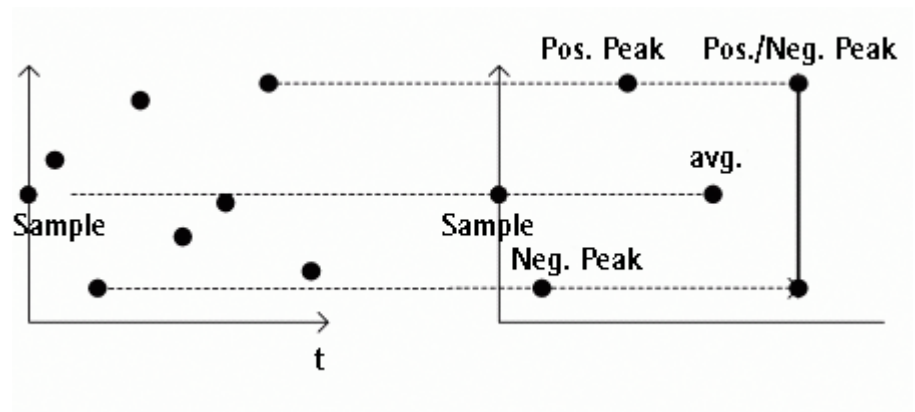
Abbildung 37 Trace-Detektoren
