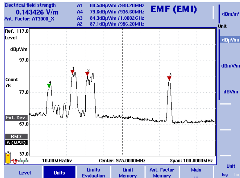
Abbildung 54 EMV-Messung
