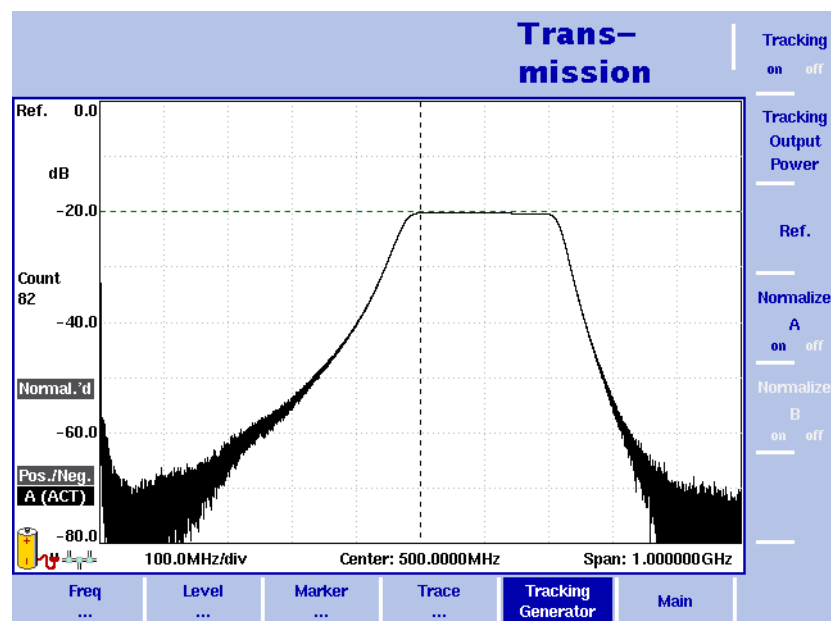
Abbildung 31 Beispiel für eine Sendemessung
