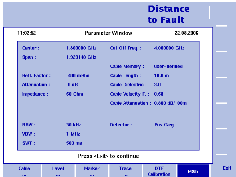
Abbildung 49 Parameter für die Kabelfehlstellenmessung
