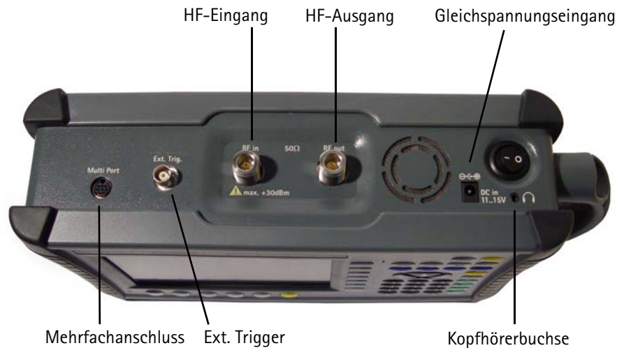
Abbildung 1 Anschlüsse 9102 an der Oberseite des Messgerätes
