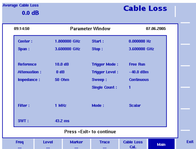
Abbildung 53 Kabeldämpfungsparameter
