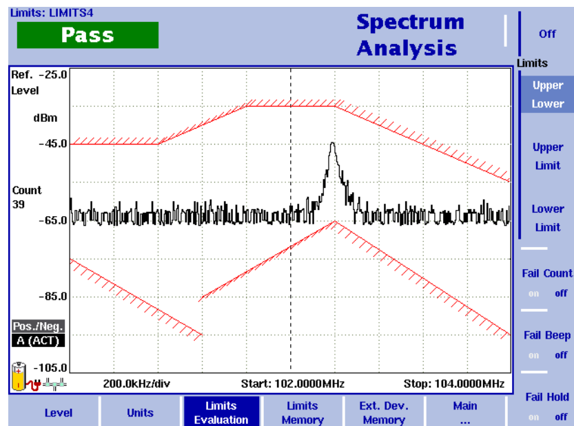
Abbildung 7 Beispiel für Begrenzungslinien bei der Spektrumanalyse
