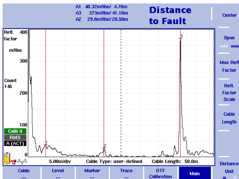
Abbildung 47 Beispiel für eine Kabelfehlstellenmessung
