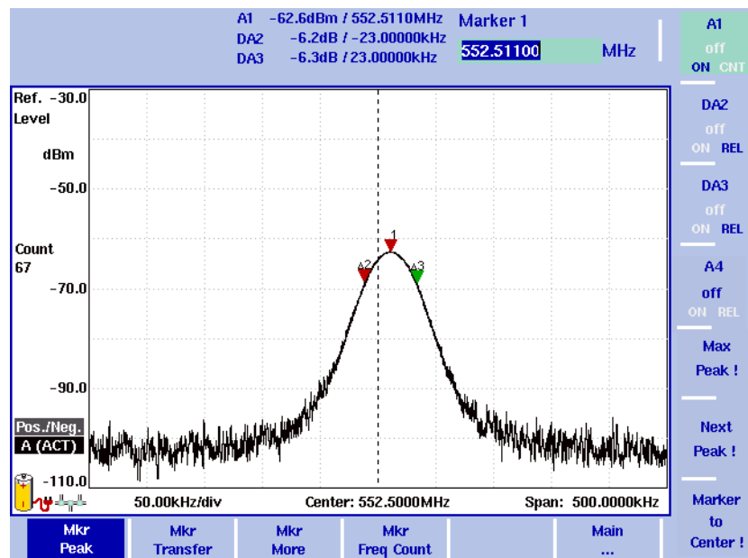
Abbildung 6 Beispiel für Marker
