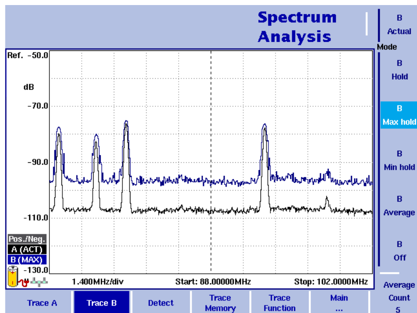
Abbildung 18 Beispiel für zwei Traces
