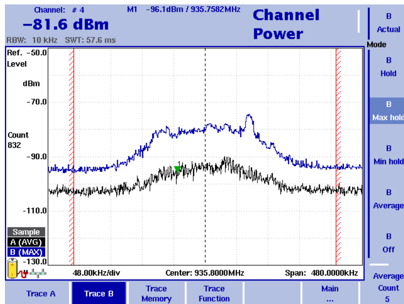
Abbildung 24 Beispiel für eine Kanalleistungsmessung
