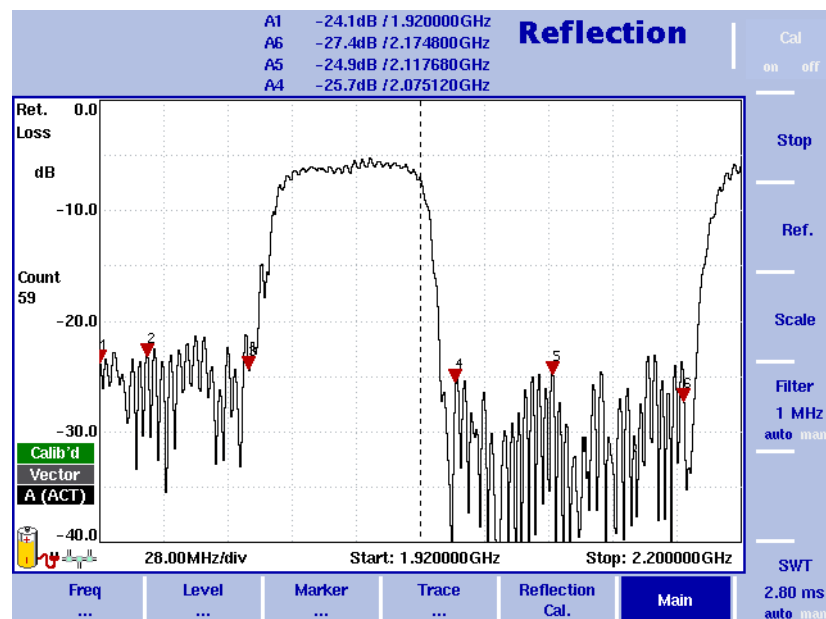
Abbildung 42 Beispiel für eine Messung der Rückflussdämpfung
